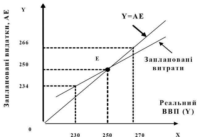
Рис. 1 – Кейнсіанський хрест
