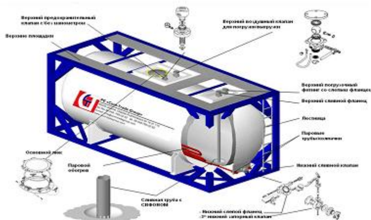
Рис. 3 – Танк-контейнер
