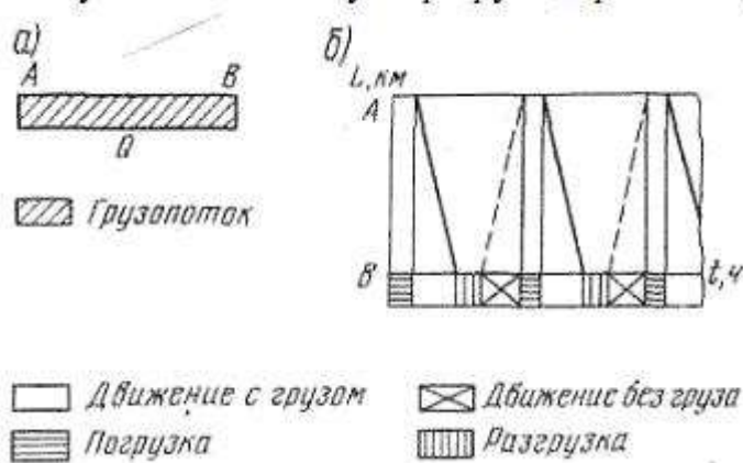
Рис. 1 – Простий маятниковий маршрут: суцільною лінією на графіку позначений пробіг з вантажем; пунктирною - пробіг без вантажу
