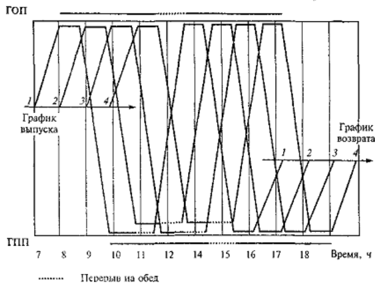
Рис. 4 – Технологічний графік роботи автотранспортних засобів
