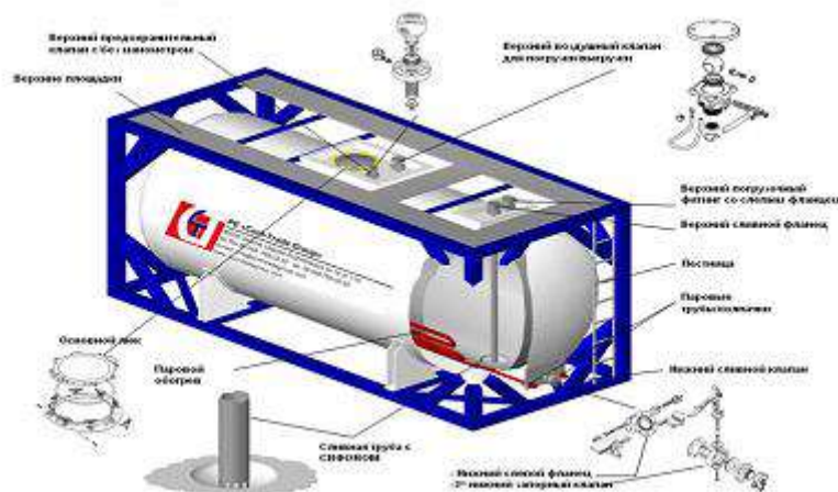
Рис. 3 – Танк-контейнер
