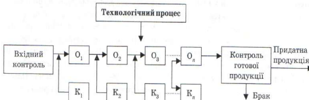
Рис. 2.2. Схема регулювання якості у процесі виробництва за допомогою статистичного контролю:
