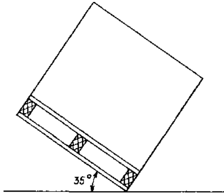
Рис. 69. Повышенная устойчивость грузового пакета, обандероленного термоусадочной пленкой
