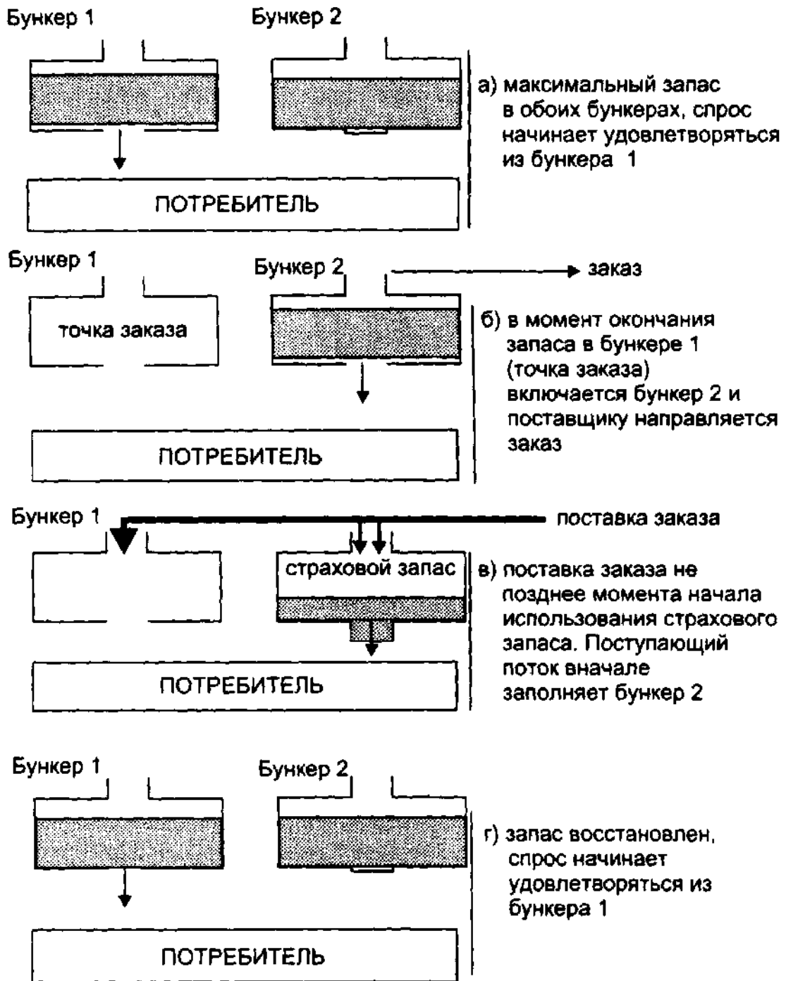
Рис. 59. Двухбункерная система контроля за состоянием запасов
